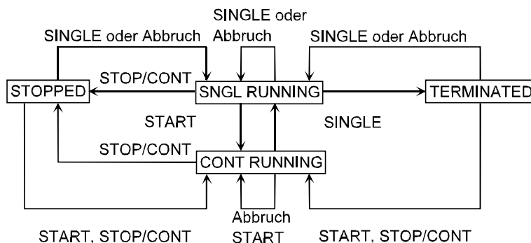
Bild 2-43 Zustandsdiagramm Meßsystem (kein Sweep aktiv)
