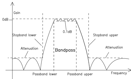
Bild 2-34 BAND PASS Frequenzgang mit Kennzeichnung der Filterparameter
