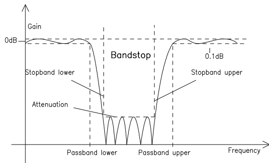
Bild 2-35 BAND STOP Frequenzgang mit Kennzeichnung der Filterparameter
